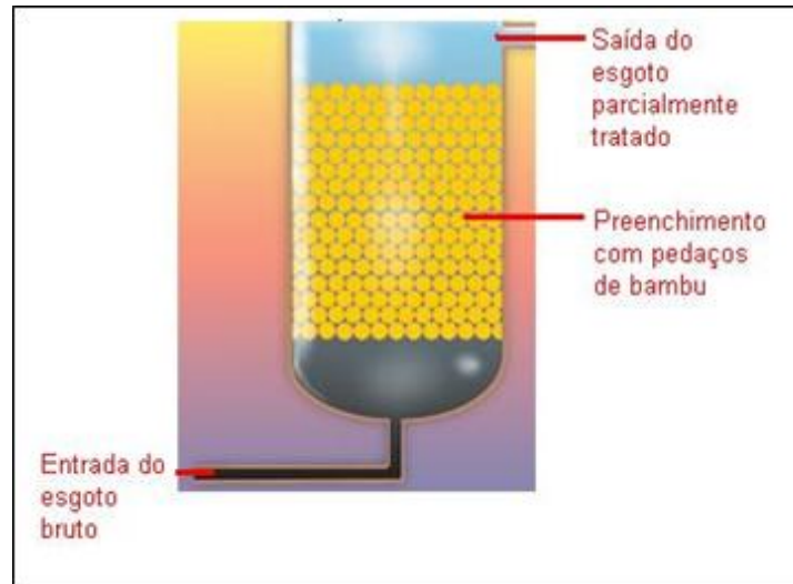
Figura 55 – Funcionamento do Reator Anaeróbico com Recheio de Bambu Fonte: Universidade Estadual de Campinas (2004)
