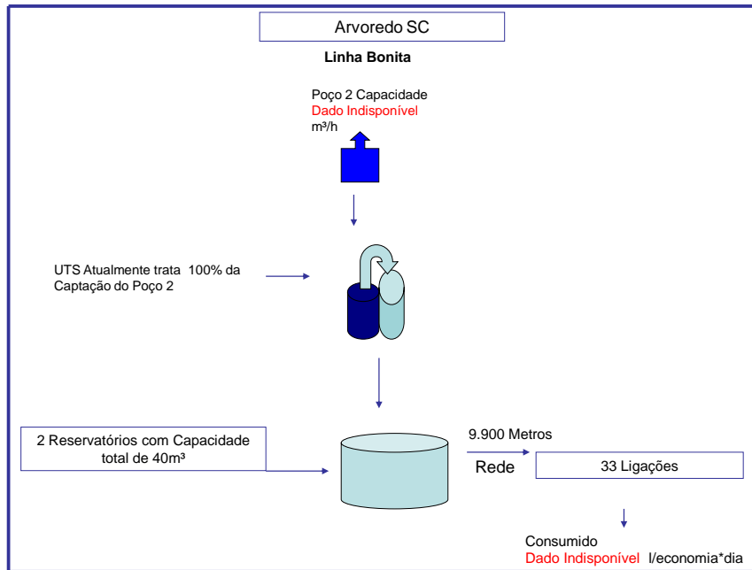
Figura 46 - Fluxograma do sistema de abastecimento de água (Linha Bonita)
