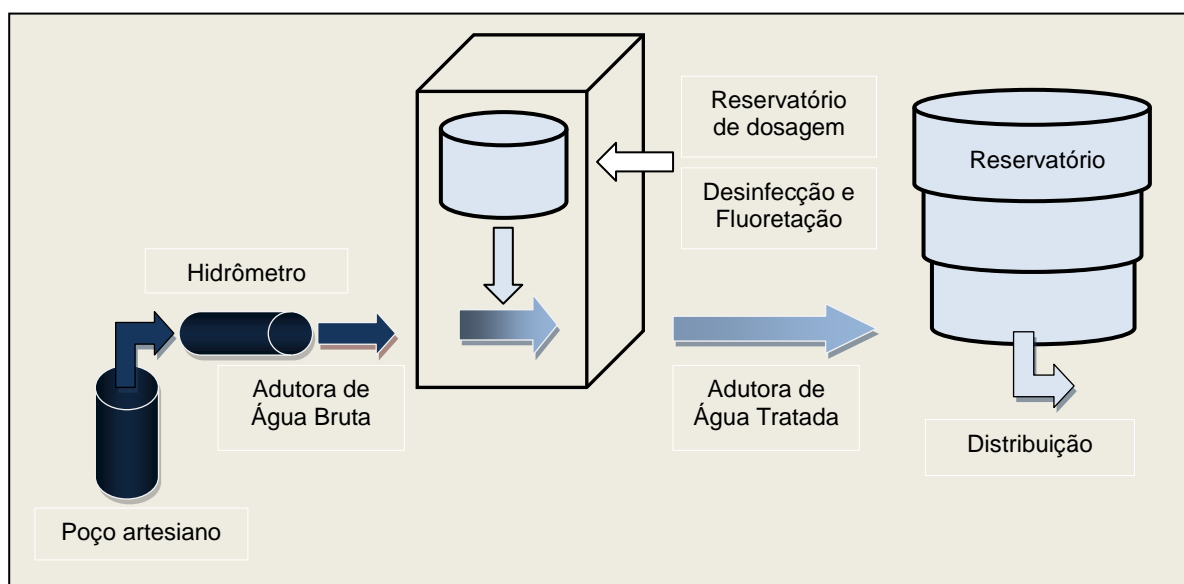
Figura 47 - Fluxograma da U.T.S.
