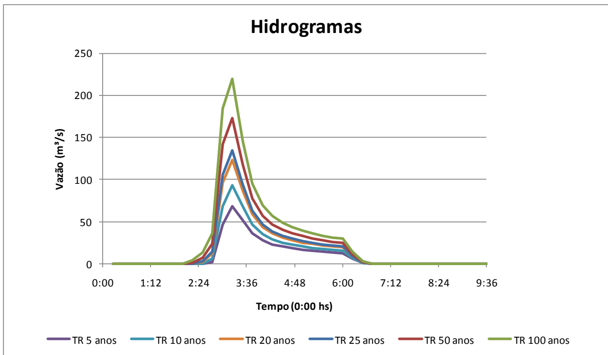
Figura 59 – Hidrogramas de Cheia
