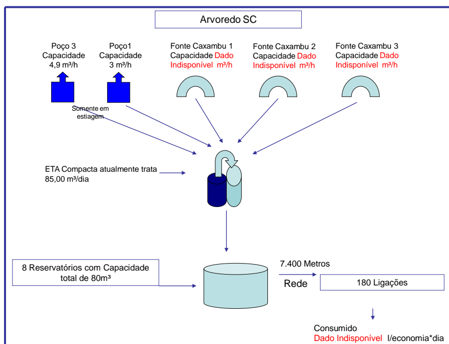
Figura 45 - Fluxograma do sistema de abastecimento de água (Sede)
