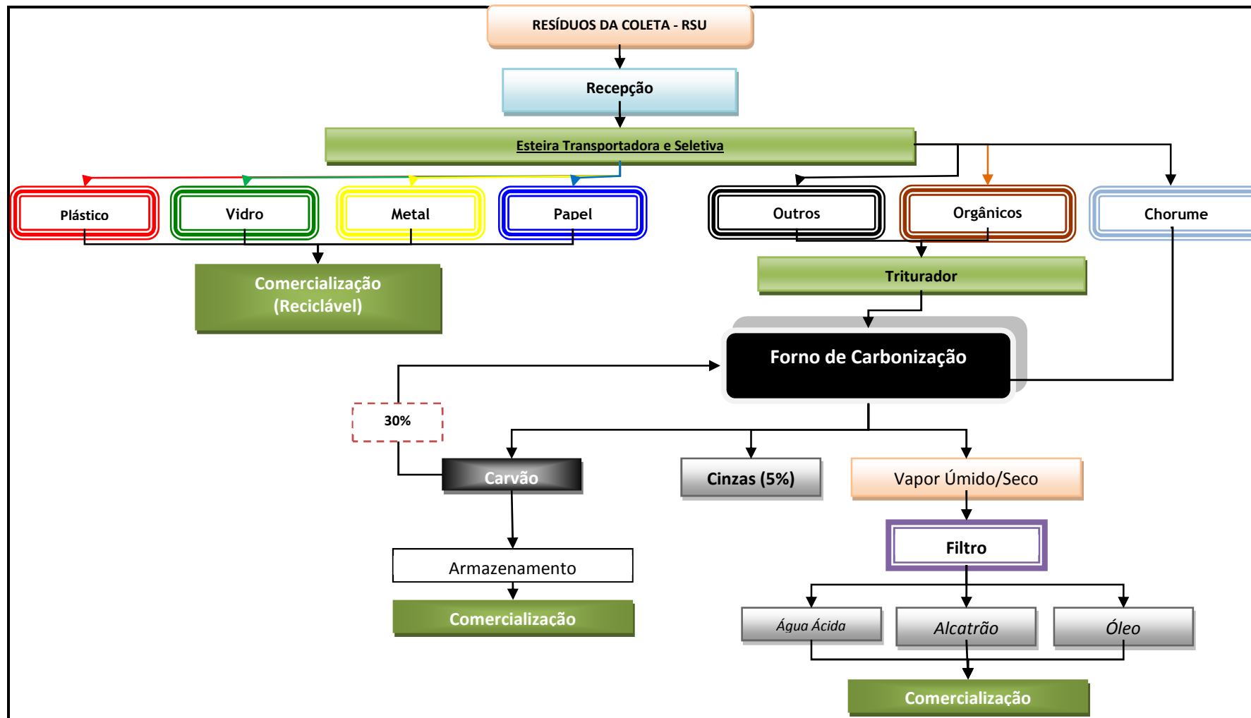
Figura 6: Fluxograma do Processo de Carbonização
