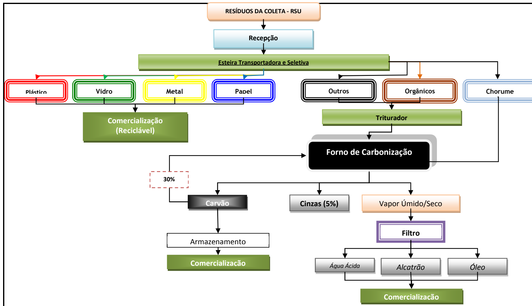
Figura 6: Fluxograma do Processo de Carbonização
